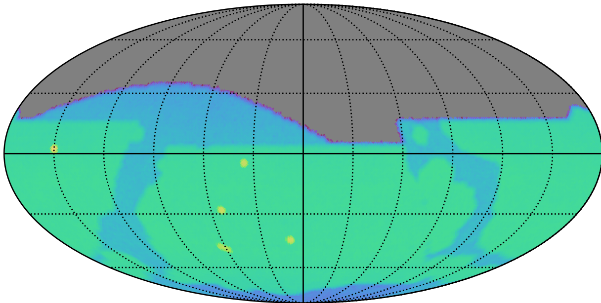
weather_cloudso6v3.4_10yrs i: SurfaceBrightLimit
