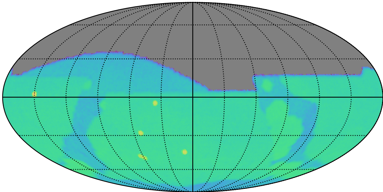
weather_cloudso6v3.4_10yrs g: SurfaceBrightLimit
