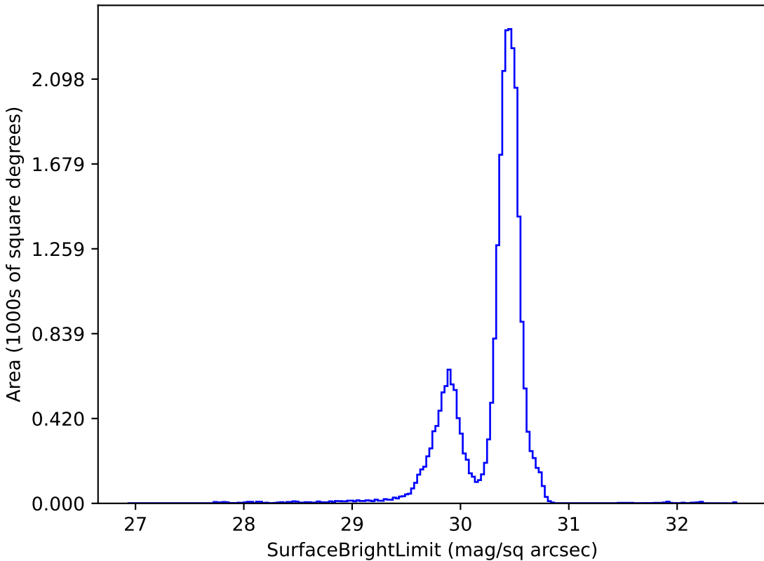
weather_cloudso6v3.4_10yrs g: SurfaceBrightLimit
