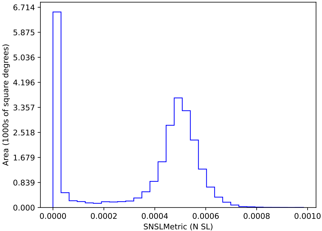
weather_cloudso6v3.4_10yrs : SNSLMetric
