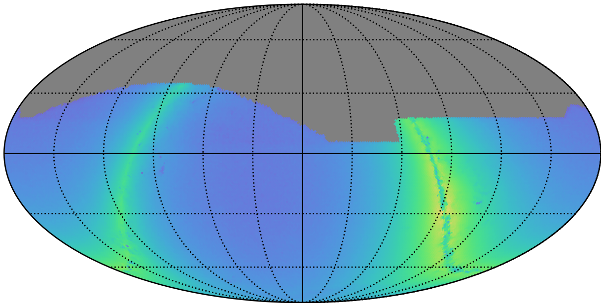
weather_cloudso6v3.4_10yrs z: Nstars_no_crowding
