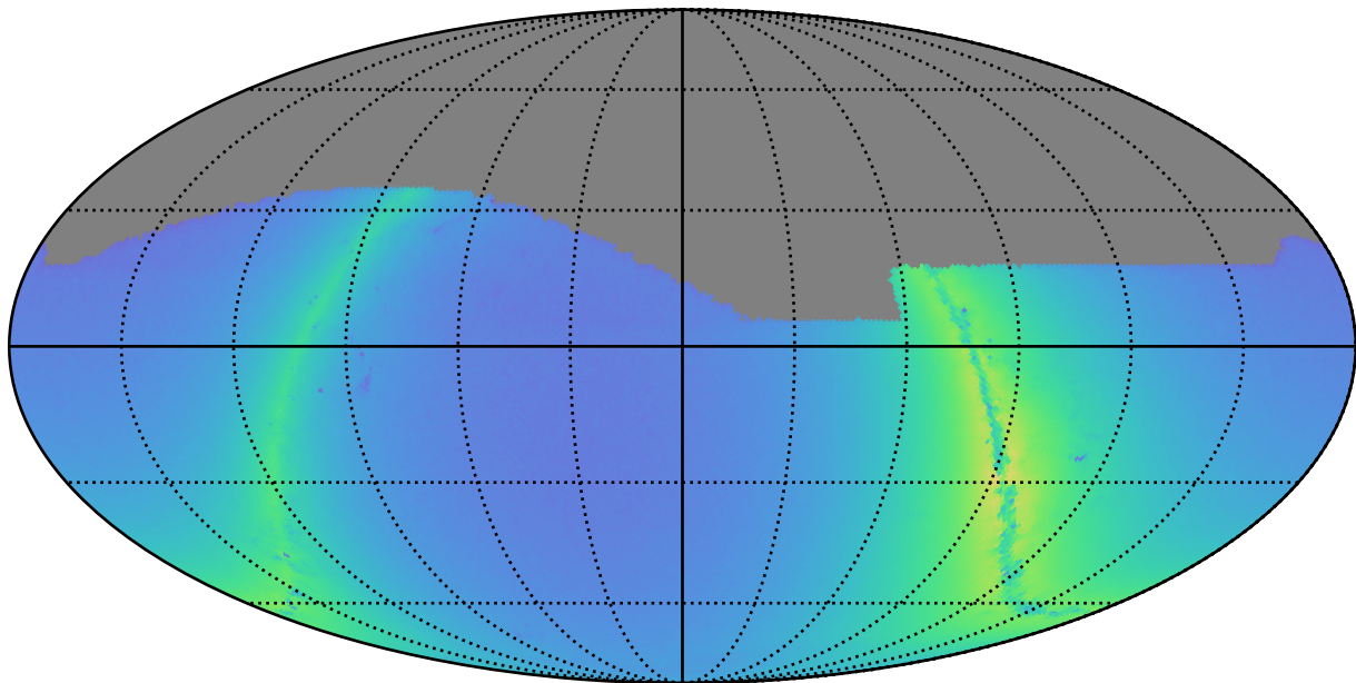
weather_cloudso6v3.4_10yrs i: Nstars_no_crowding
