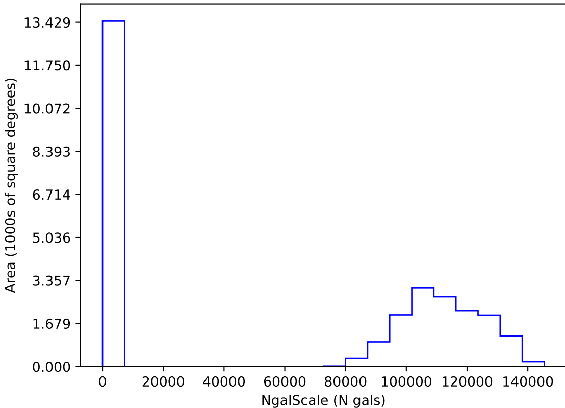
weather_cloudso6v3.4_10yrs i: NgalScale
