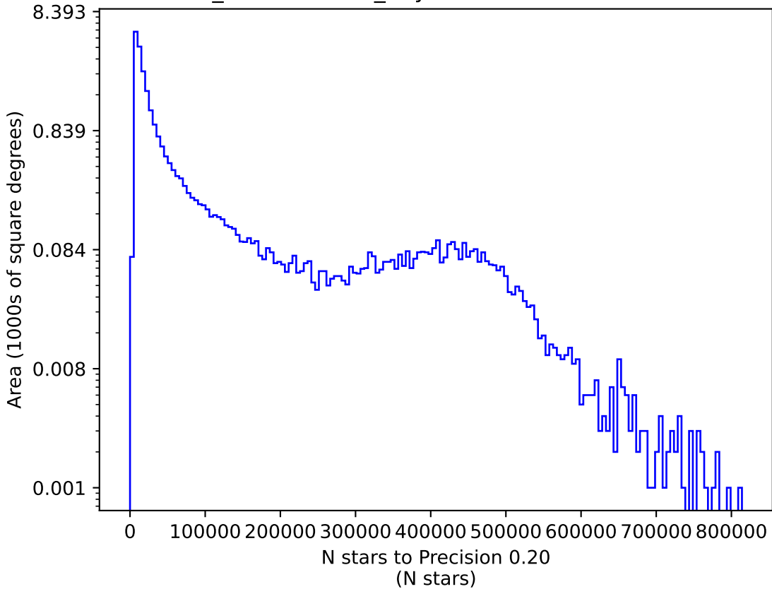
weather_cloudso6v3.4_10yrs i: N stars to Precision 0.20
