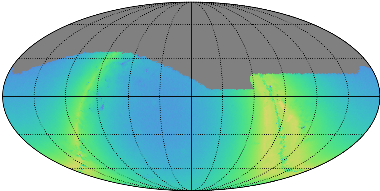
weather_cloudso6v3.4_10yrs g: N stars to Precision 0.20
