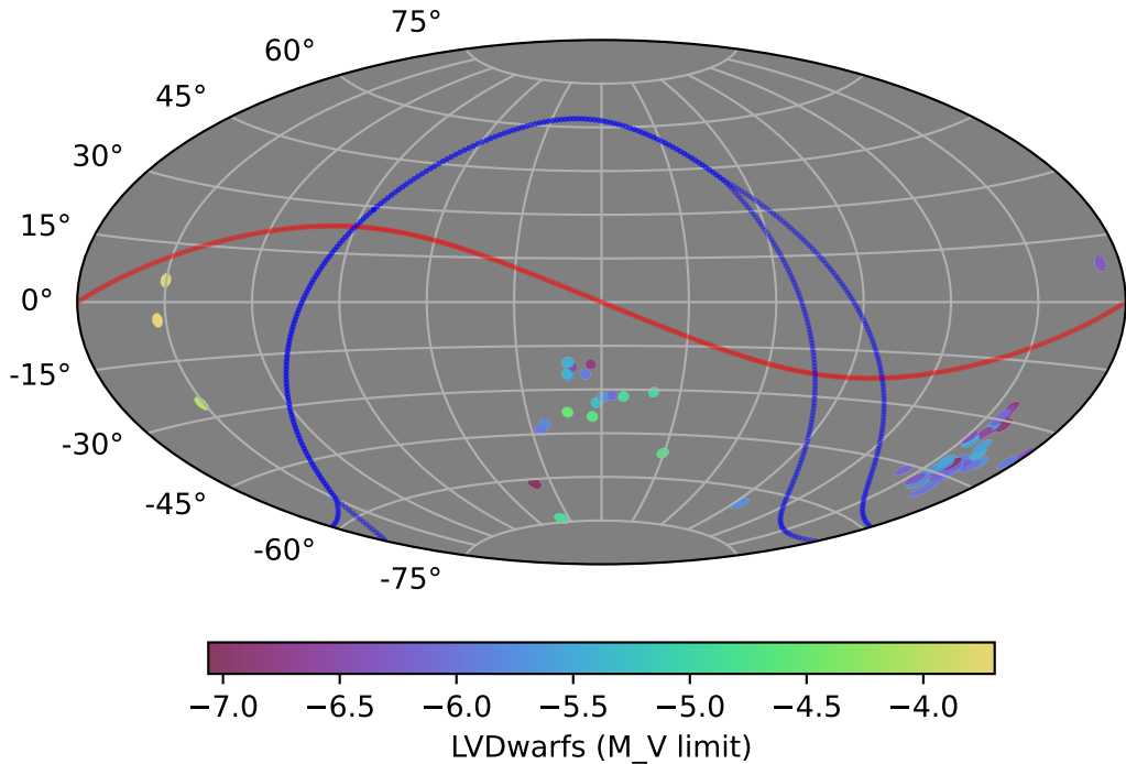
weather_cloudso6v3.4_10yrs gi: LVDwarfs
