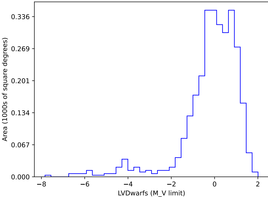
weather_cloudso6v3.4_10yrs gi SCP: LVDwarfs
