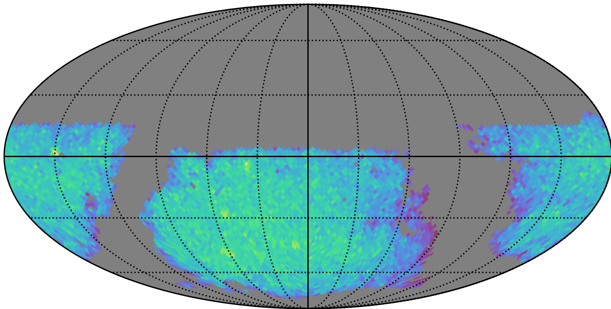
weather_cloudso6v3.4_10yrs gi: LVDwarfs
