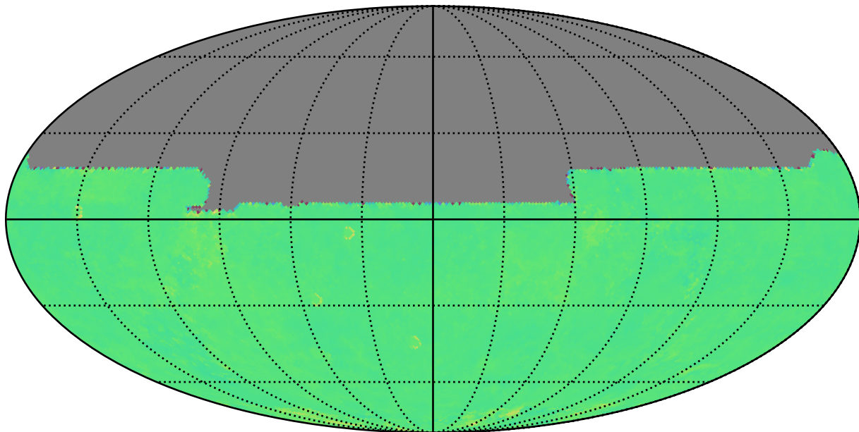
weather_cloudso6v3.4_10yrs y: Kuiper rotTelPos
