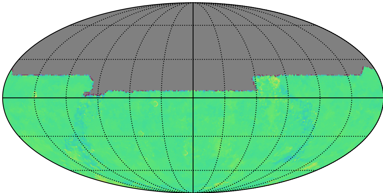
weather_cloudso6v3.4_10yrs u: Kuiper rotTelPos
