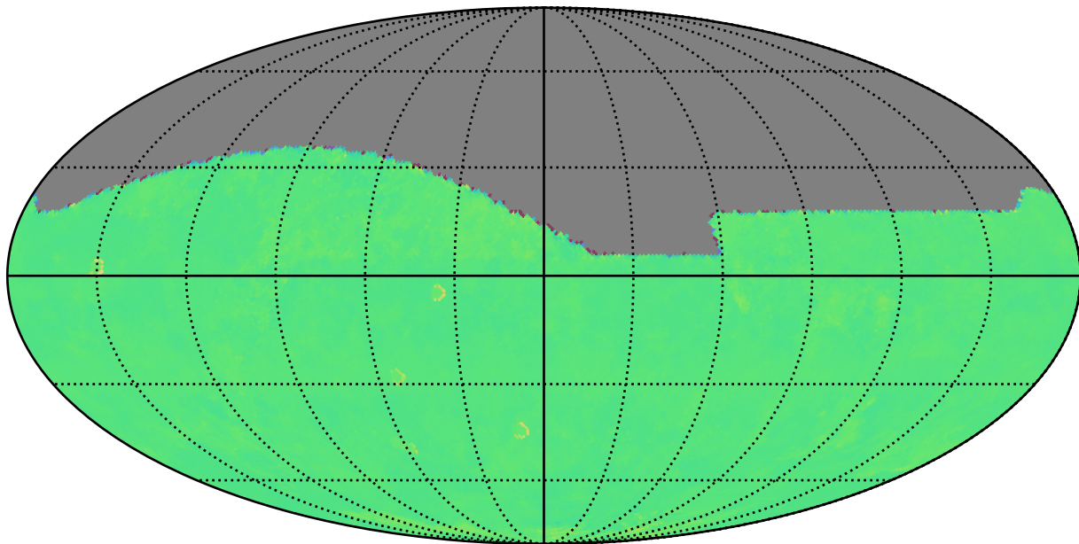
weather_cloudso6v3.4_10yrs i: Kuiper rotTelPos
