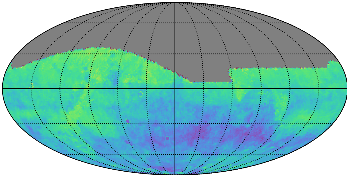
weather_cloudso6v3.4_10yrs z: Kuiper rotSkyPos
