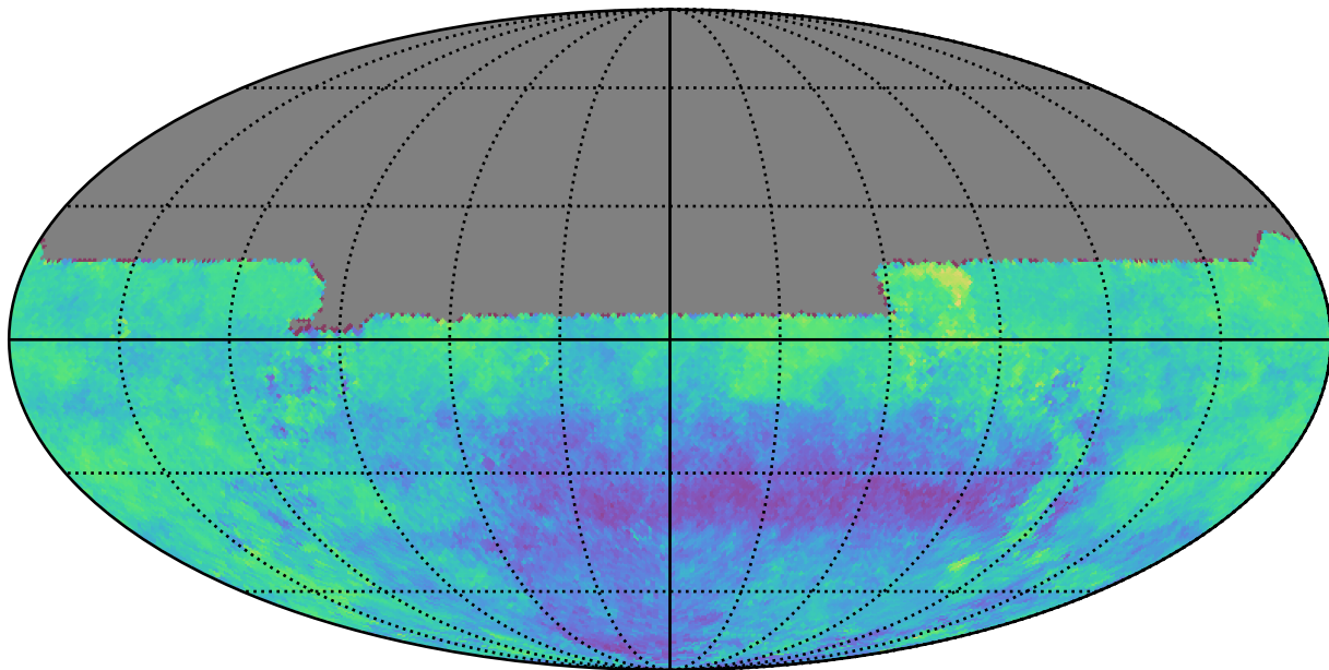
weather_cloudso6v3.4_10yrs u: Kuiper rotSkyPos
