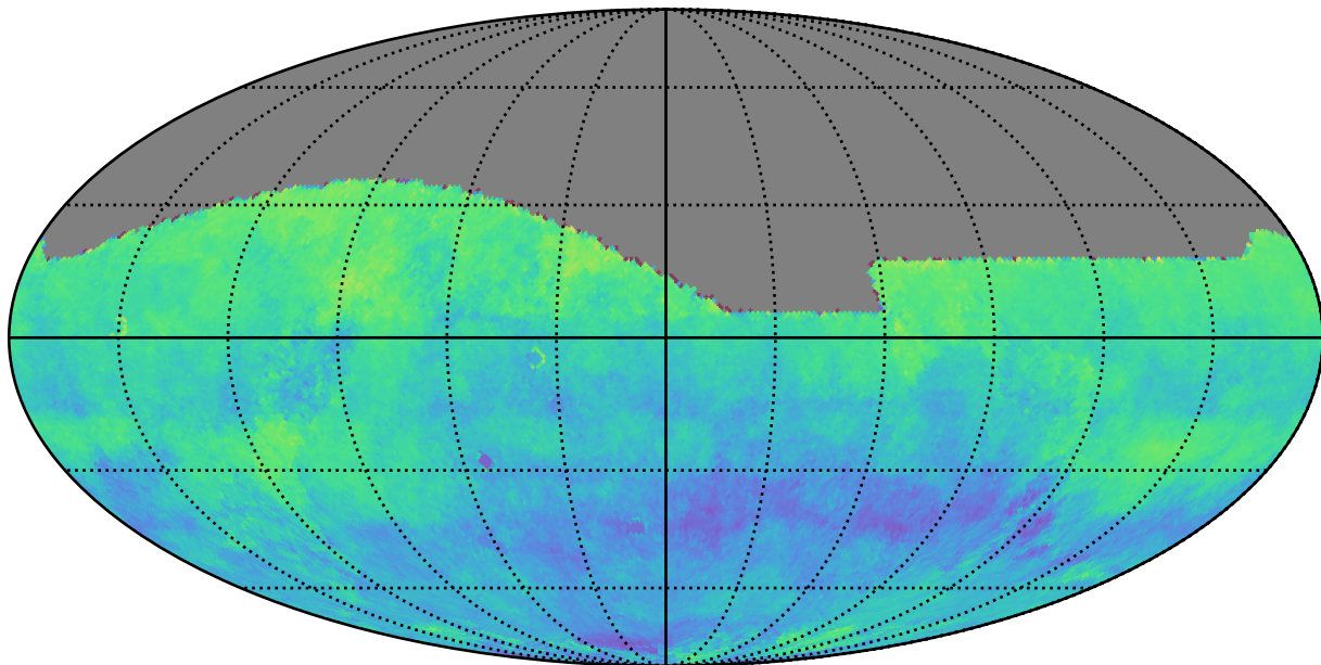
weather_cloudso6v3.4_10yrs i: Kuiper rotSkyPos
