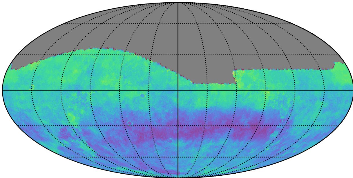
weather_cloudso6v3.4_10yrs g: Kuiper rotSkyPos
