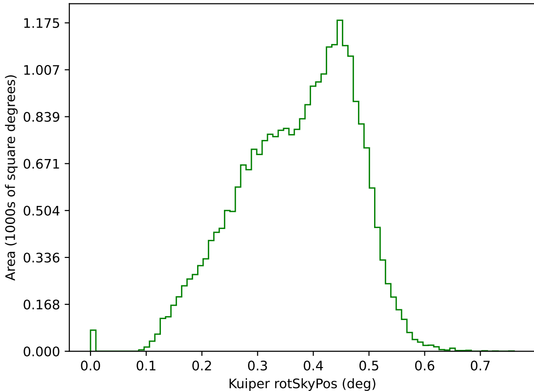
weather_cloudso6v3.4_10yrs g: Kuiper rotSkyPos
