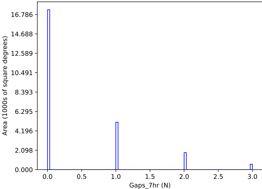
weather_cloudso6v3.4_10yrs y band: Gaps_7hr
