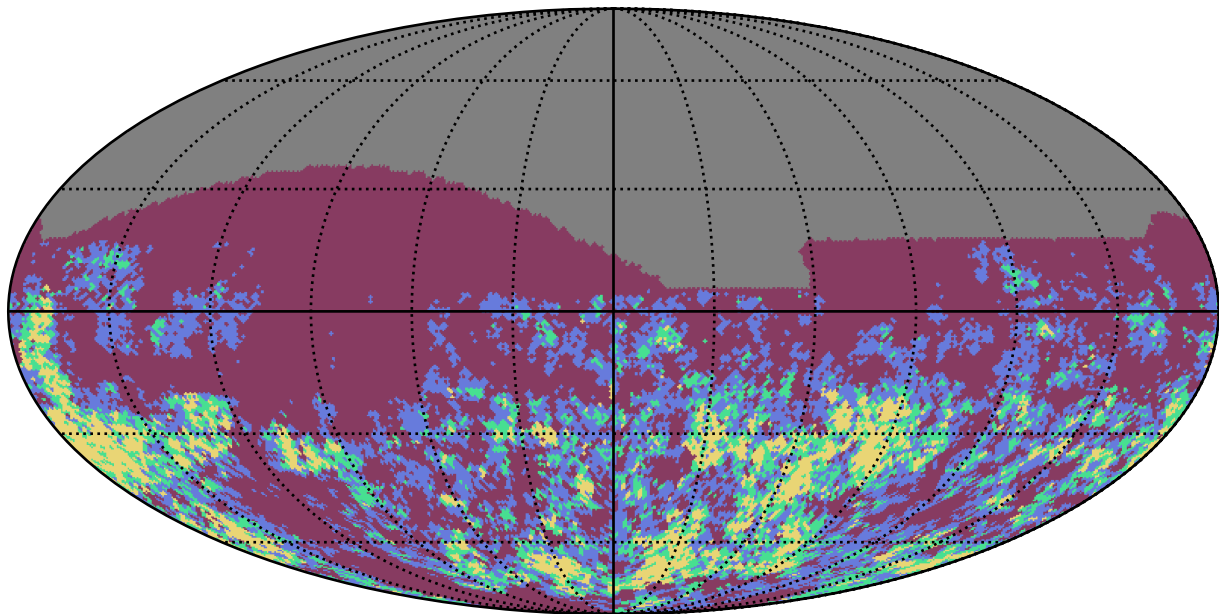
weather_cloudso6v3.4_10yrs i band: Gaps_7hr
