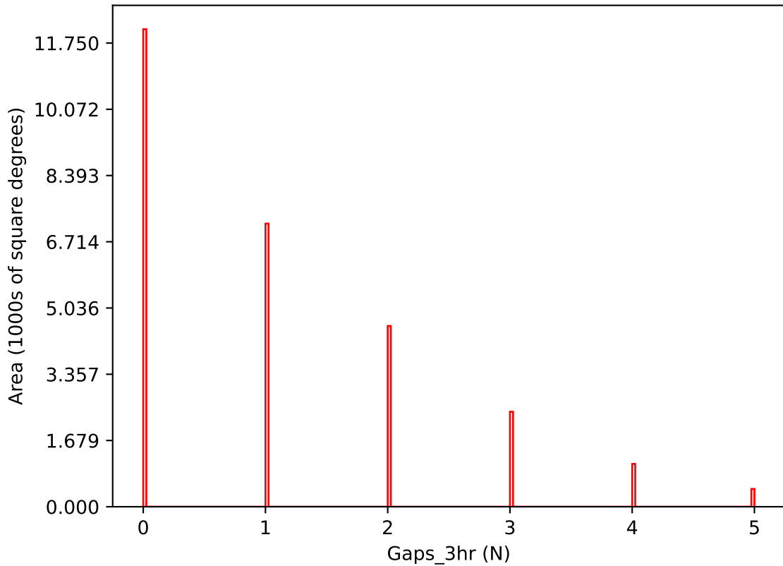
weather_cloudso6v3.4_10yrs i band: Gaps_3hr
