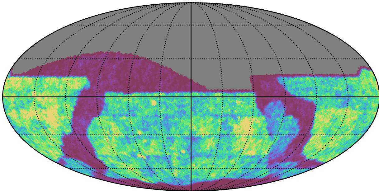
weather_cloudso6v3.4_10yrs z band: Gaps_24hr
