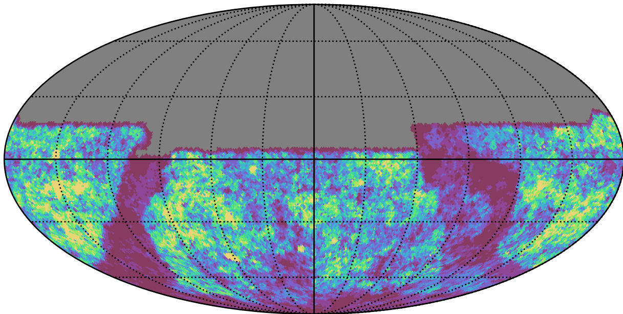
weather_cloudso6v3.4_10yrs u band: Gaps_24hr
