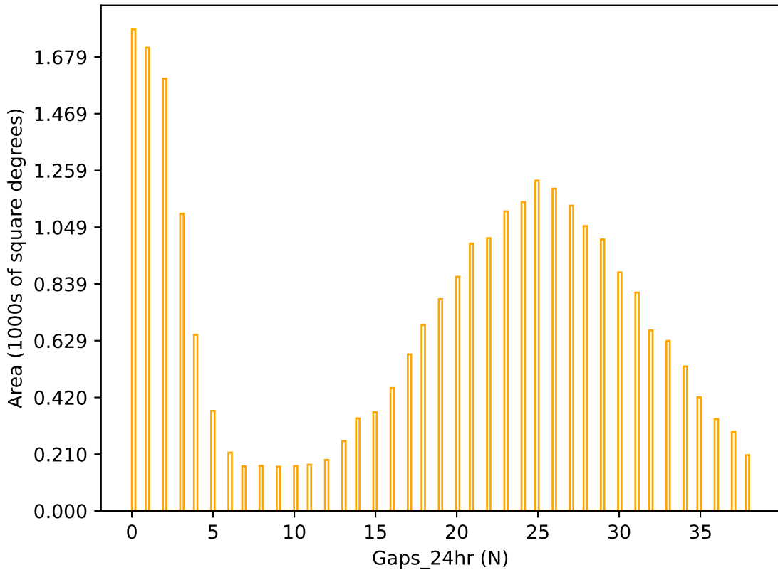
weather_cloudso6v3.4_10yrs r band: Gaps_24hr
