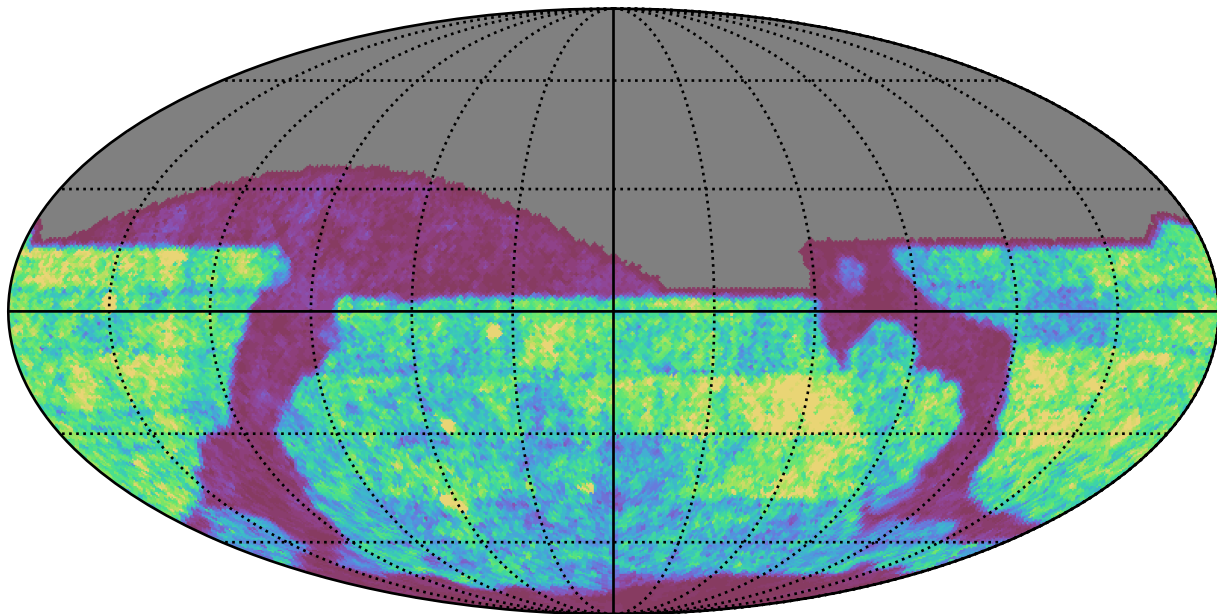
weather_cloudso6v3.4_10yrs i band: Gaps_24hr
