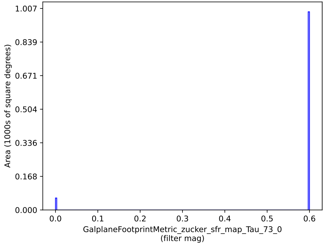
weather_cloudso6v3.4_10yrs : GalplaneFootprintMetric_zucker_sfr_map_Tau_73_0
