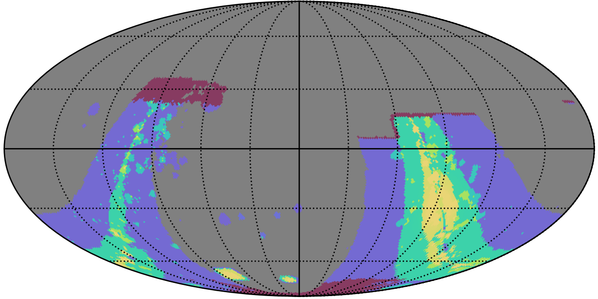
weather_cloudso6v3.4_10yrs : GalplaneFootprintMetric_combined_map_Tau_46_5
