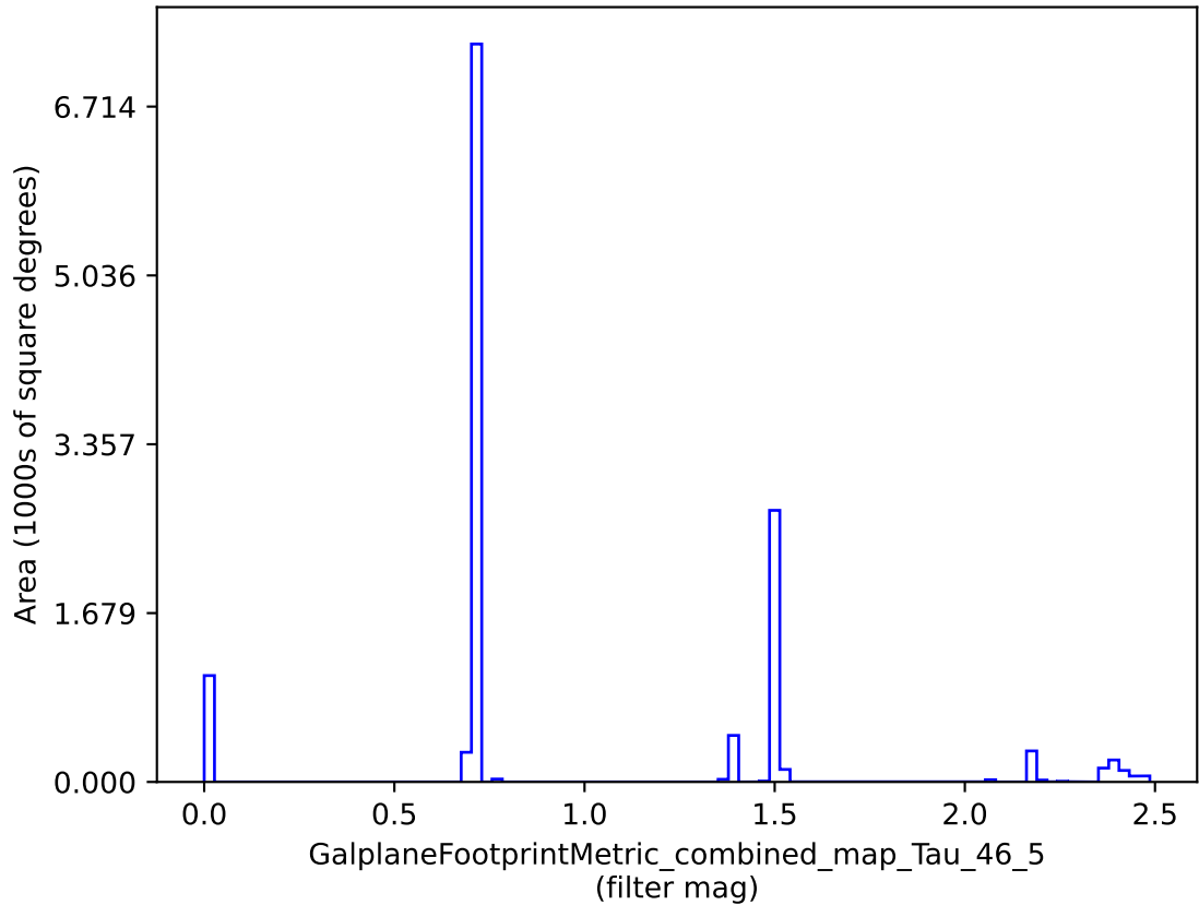
weather_cloudso6v3.4_10yrs : GalplaneFootprintMetric_combined_map_Tau_46_5
