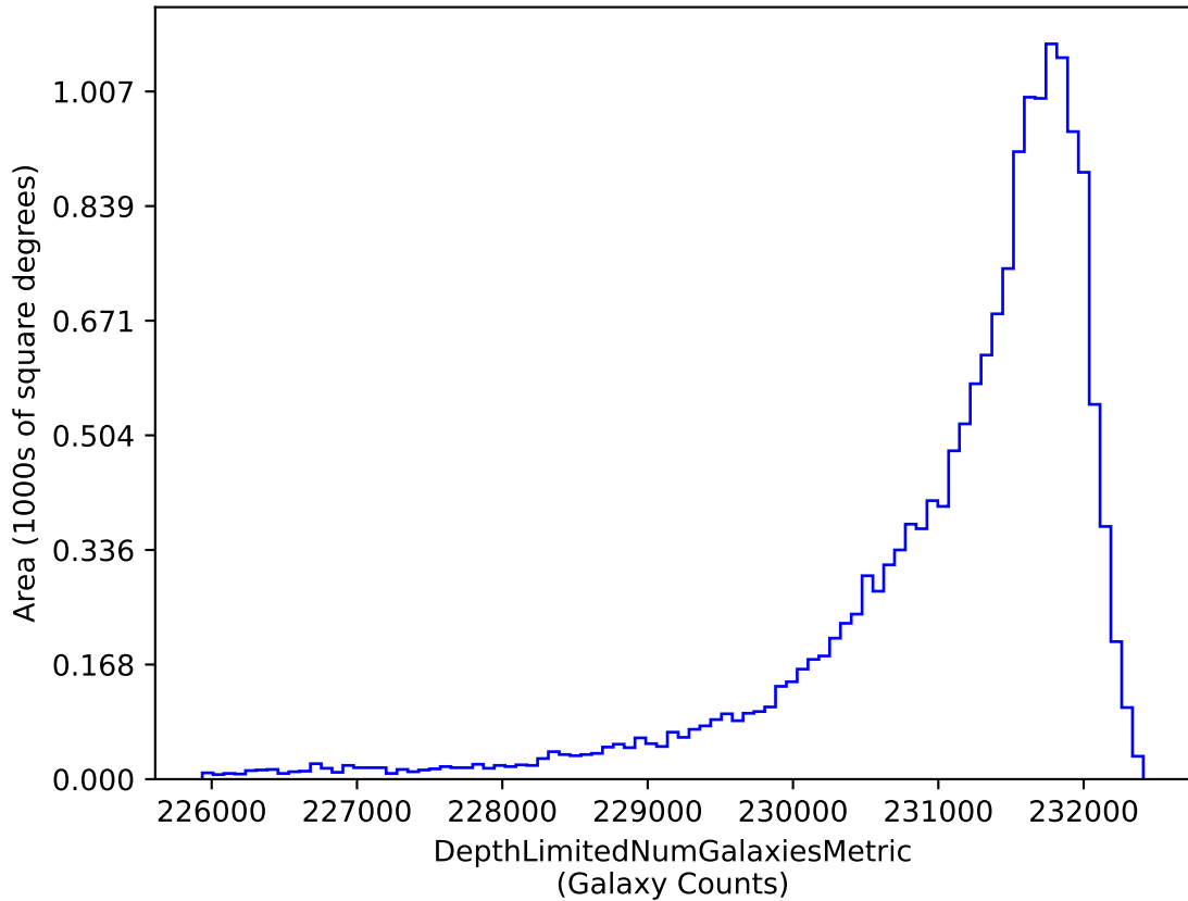
weather_cloudso6v3.4_10yrs i band galaxies non-DD: DepthLimitedNumGalaxiesMetric
