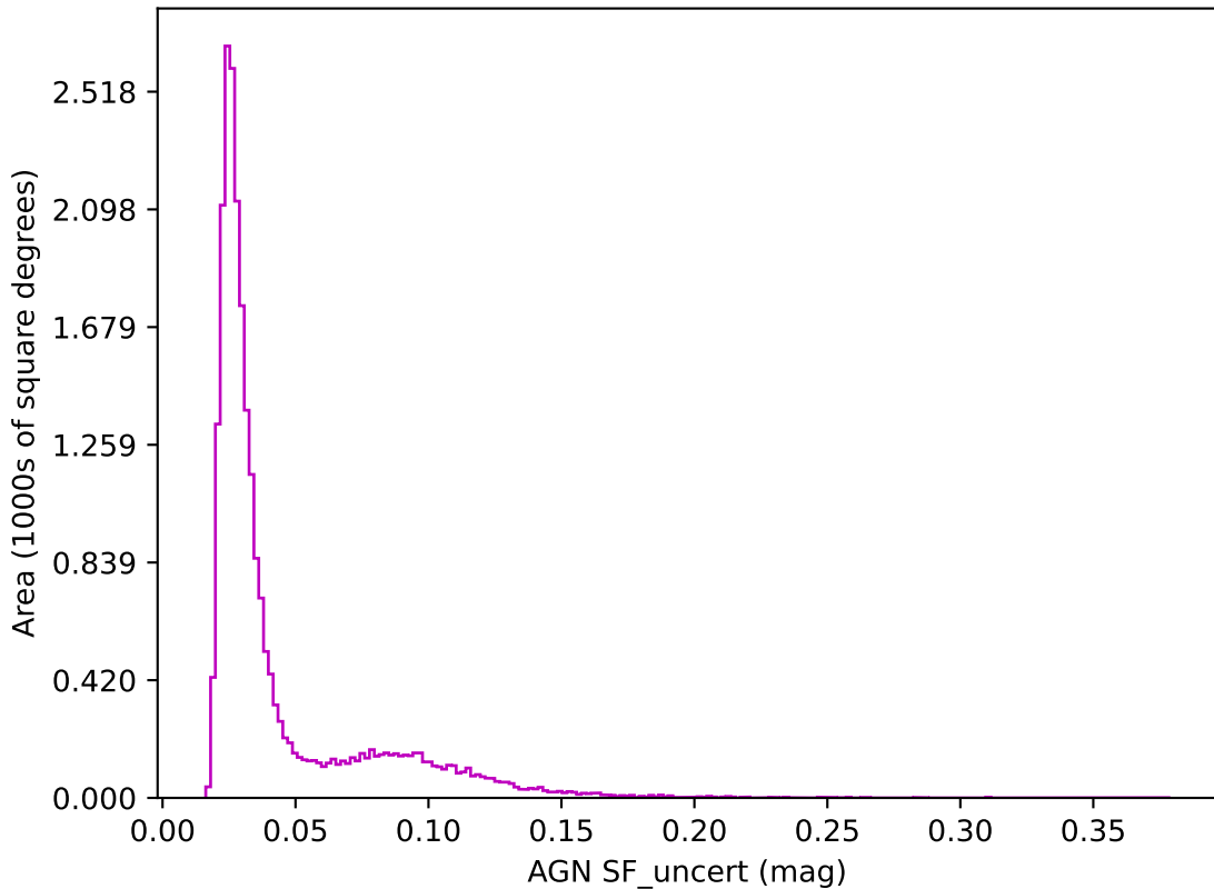
weather_cloudso6v3.4_10yrs z band: AGN SF_uncert
