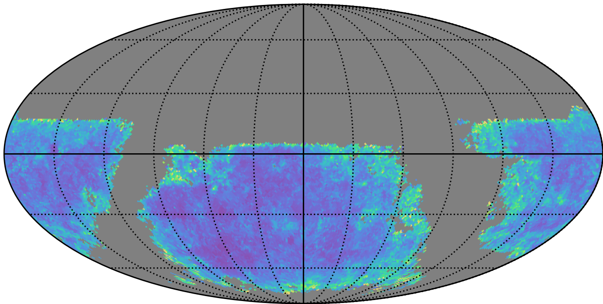
weather_cloudso6v3.4_10yrs u band: AGN SF_uncert
