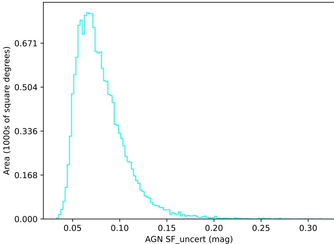
weather_cloudso6v3.4_10yrs u band: AGN SF_uncert
