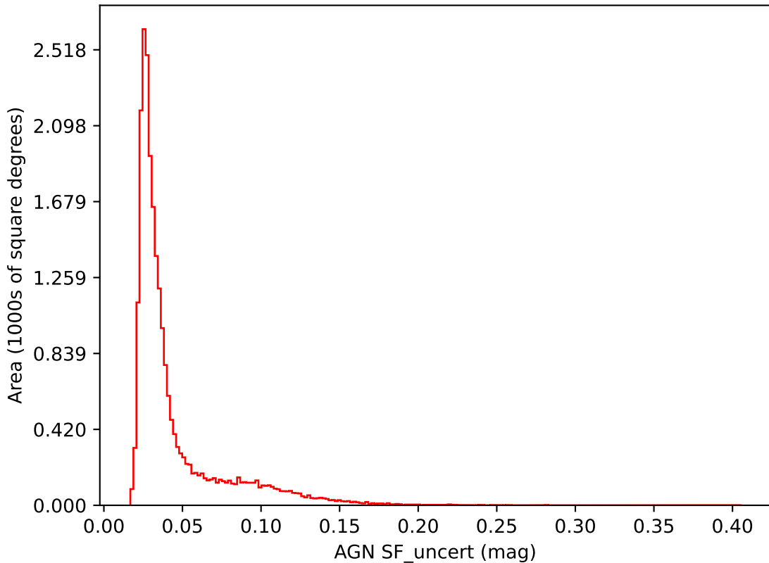
weather_cloudso6v3.4_10yrs i band: AGN SF_uncert
