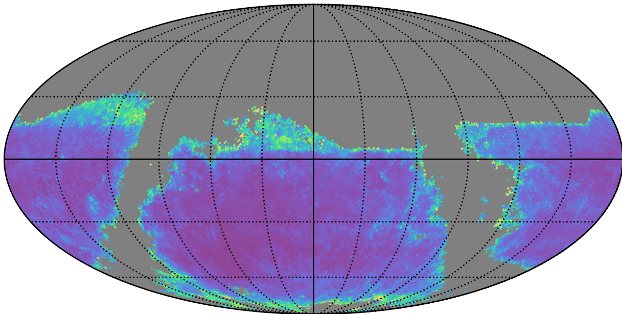
weather_cloudso6v3.4_10yrs g band: AGN SF_uncert
