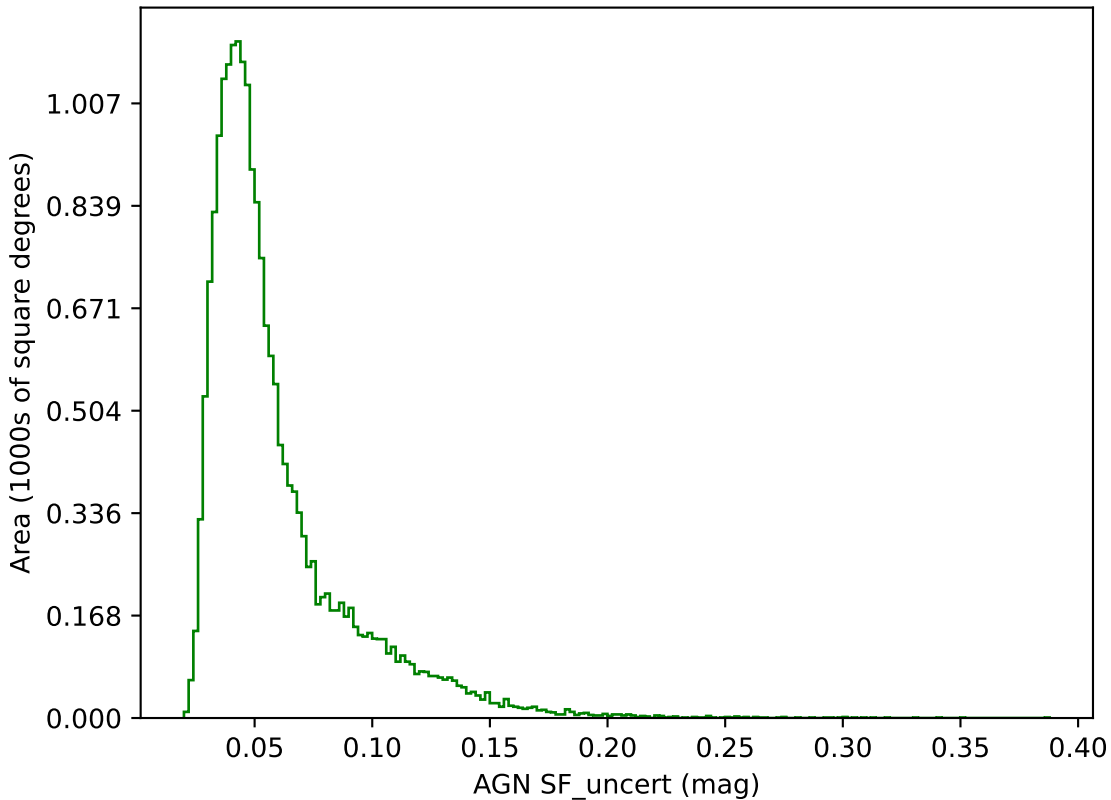
weather_cloudso6v3.4_10yrs g band: AGN SF_uncert
