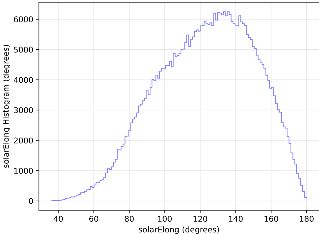
weather_cloudso6v3.4_10yrs WFD y band: solarElong Histogram
