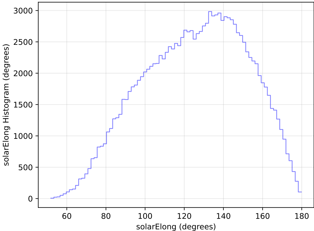
weather_cloudso6v3.4_10yrs WFD u band: solarElong Histogram
