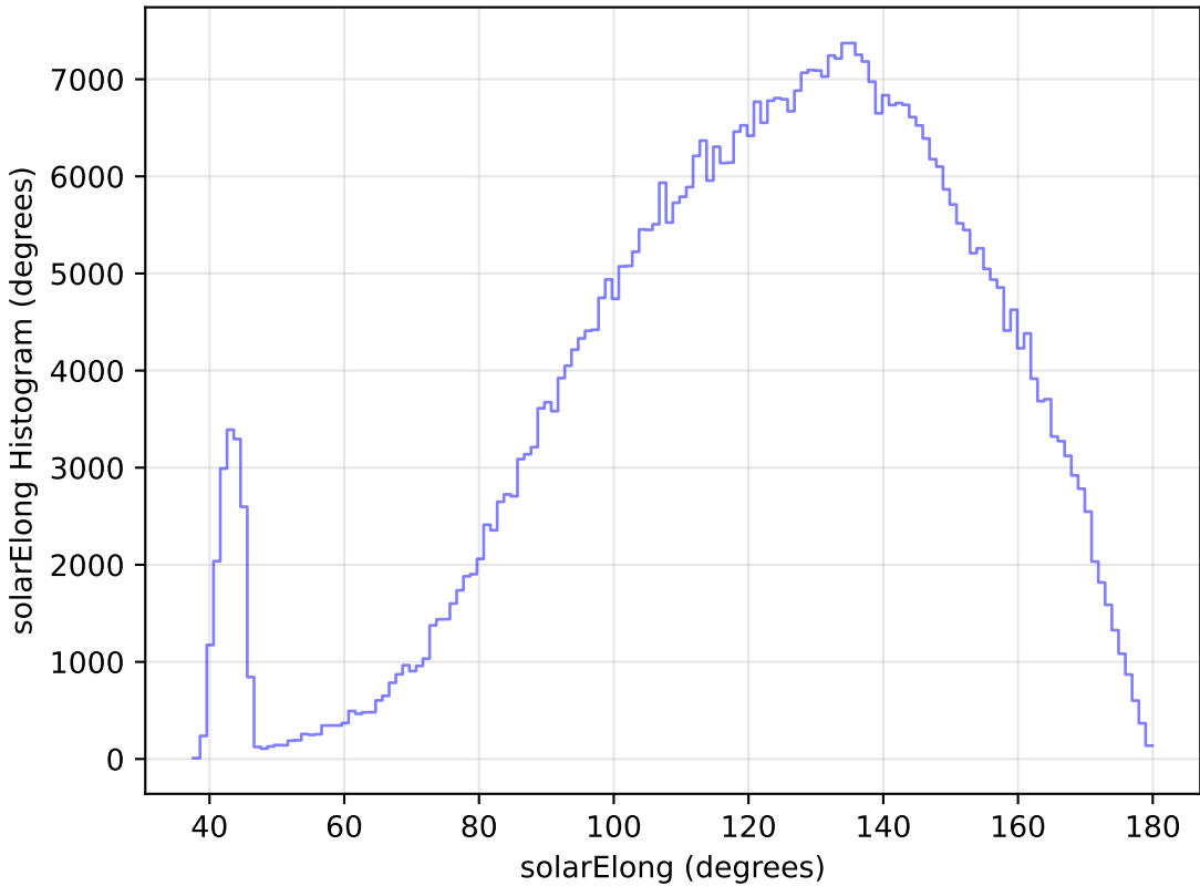
weather_cloudso6v3.4_10yrs WFD r band: solarElong Histogram
