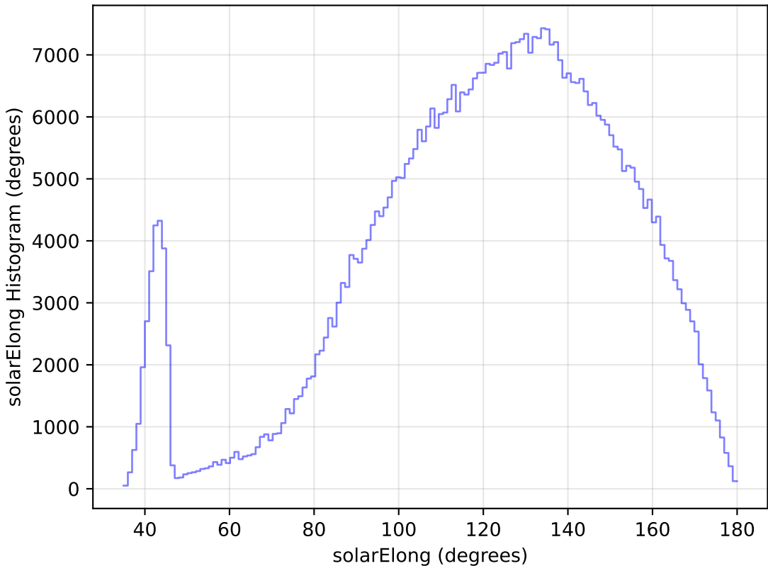
weather_cloudso6v3.4_10yrs WFD i band: solarElong Histogram
