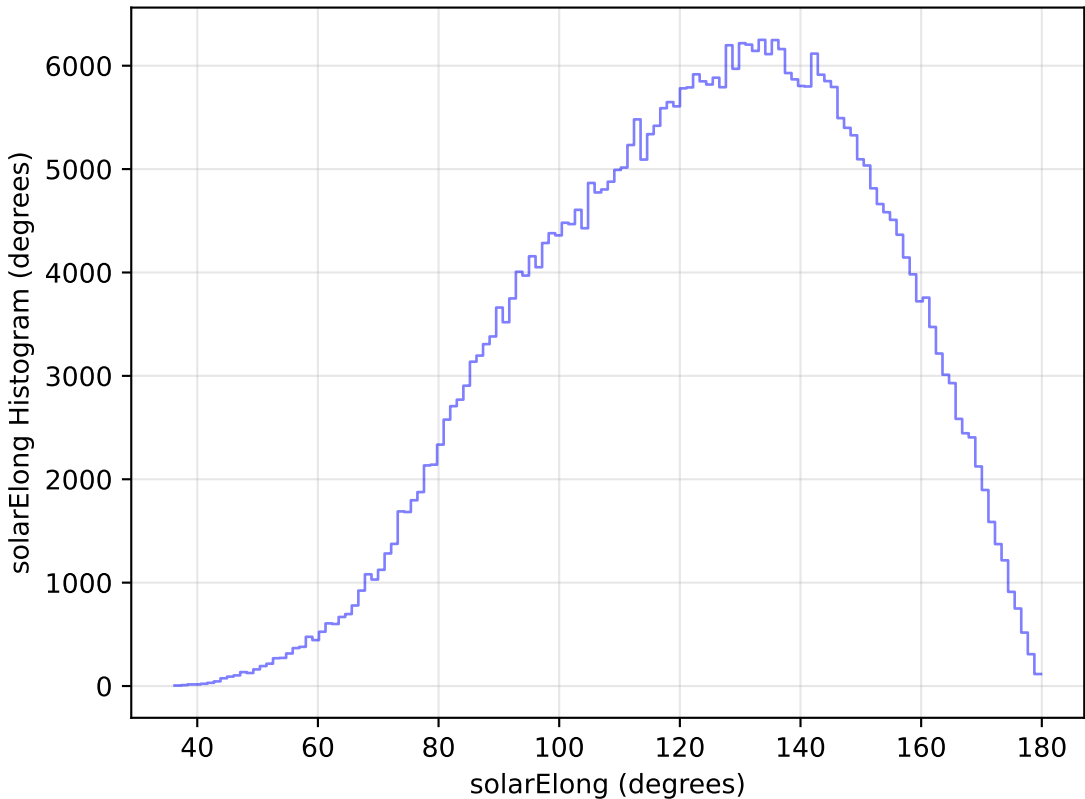
weather_cloudso6v3.4_10yrs All sky y band: solarElong Histogram
