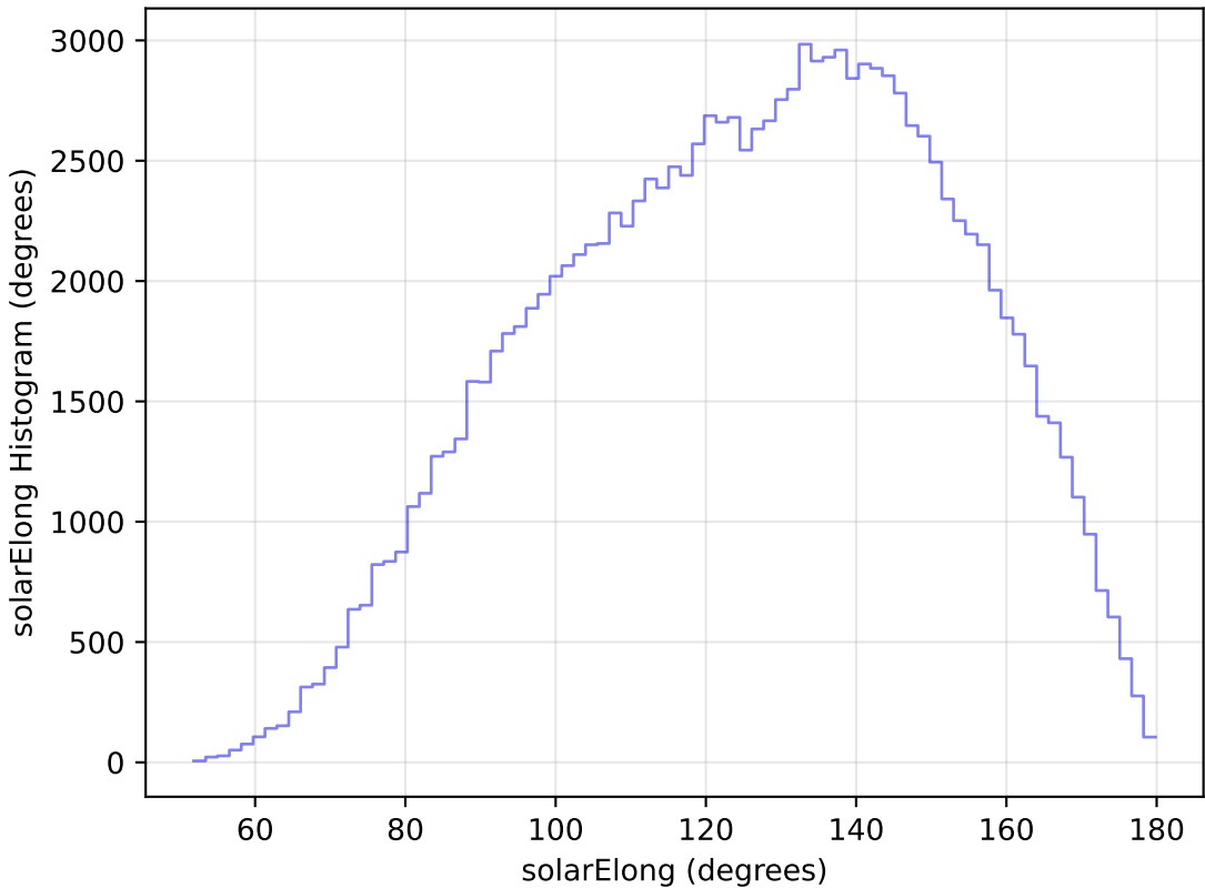
weather_cloudso6v3.4_10yrs All sky u band: solarElong Histogram
