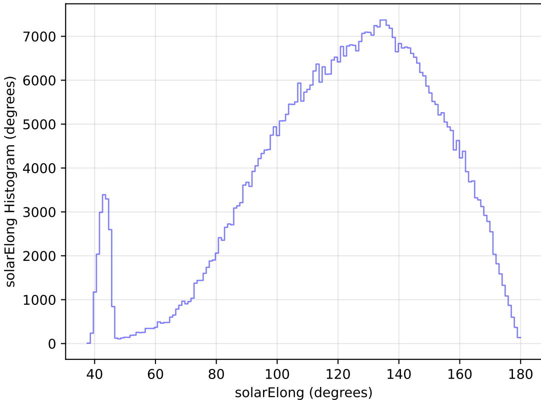
weather_cloudso6v3.4_10yrs All sky r band: solarElong Histogram
