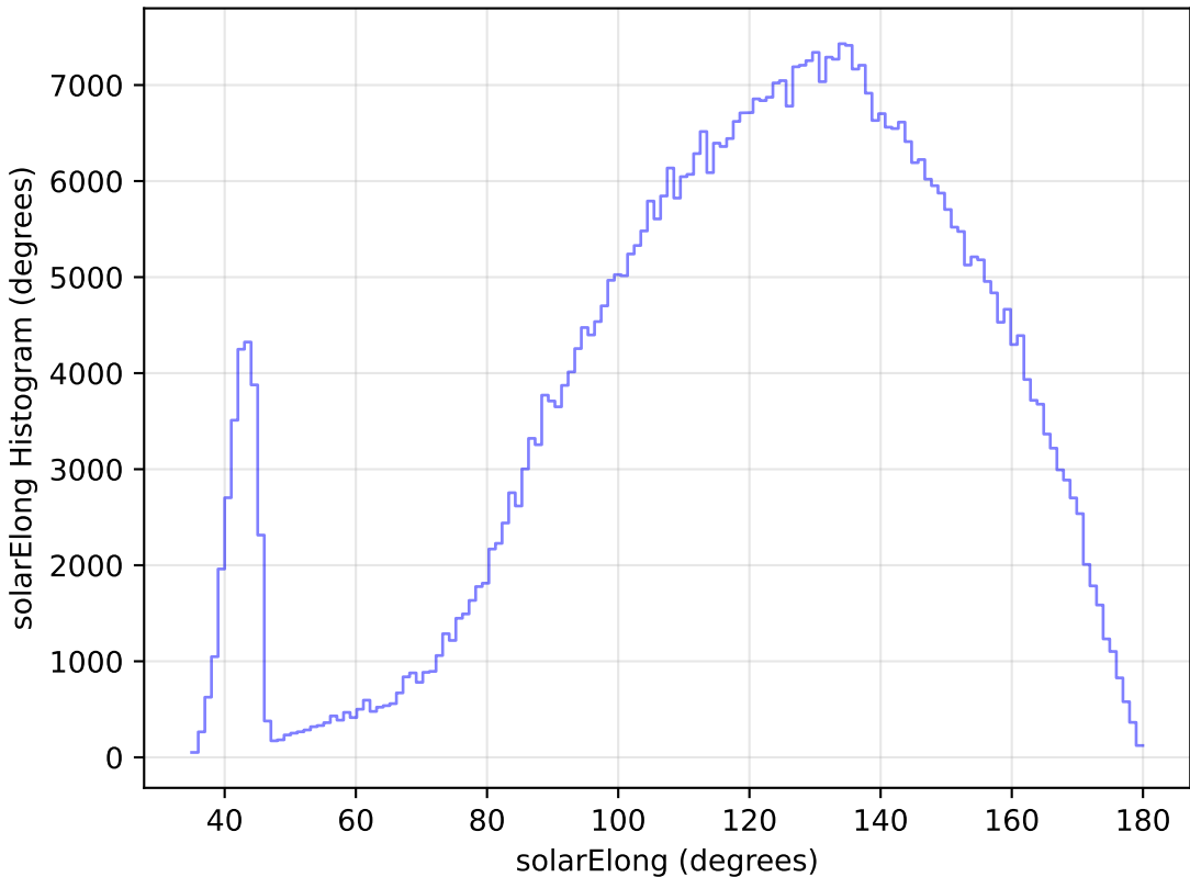
weather_cloudso6v3.4_10yrs All sky i band: solarElong Histogram
