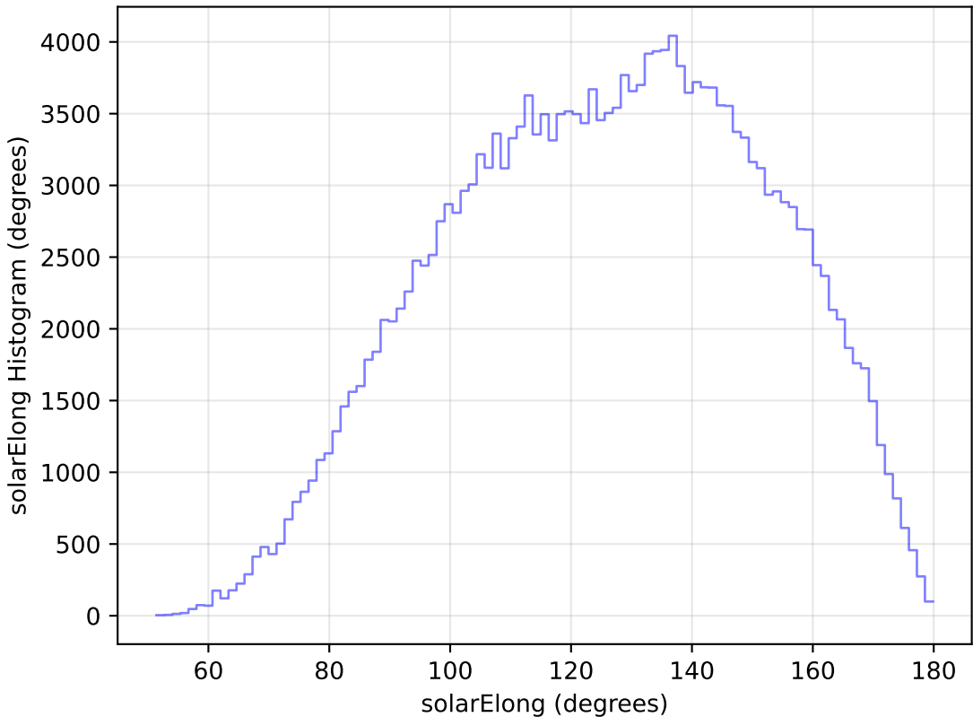
weather_cloudso6v3.4_10yrs All sky g band: solarElong Histogram
