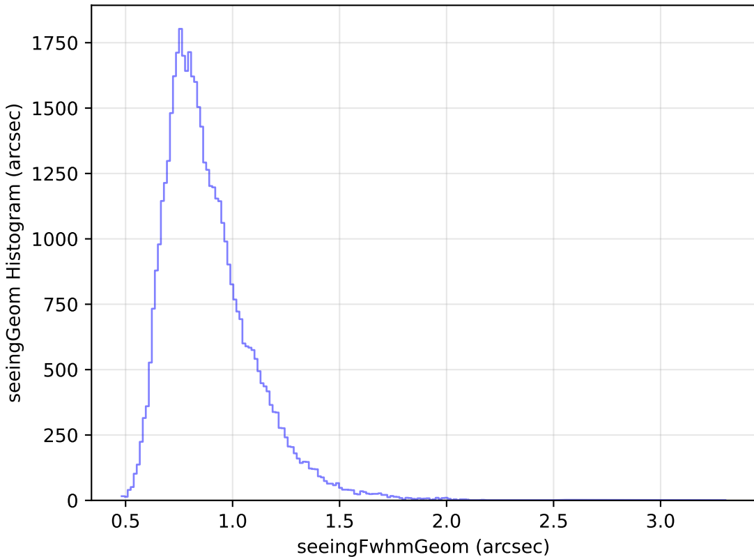
weather_cloudso6v3.4_10yrs Yr 1 y band: seeingGeom Histogram
