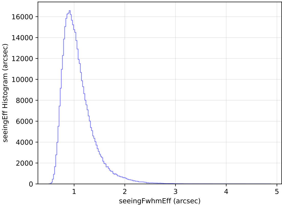
weather_cloudso6v3.4_10yrs WFD y band: seeingEff Histogram
