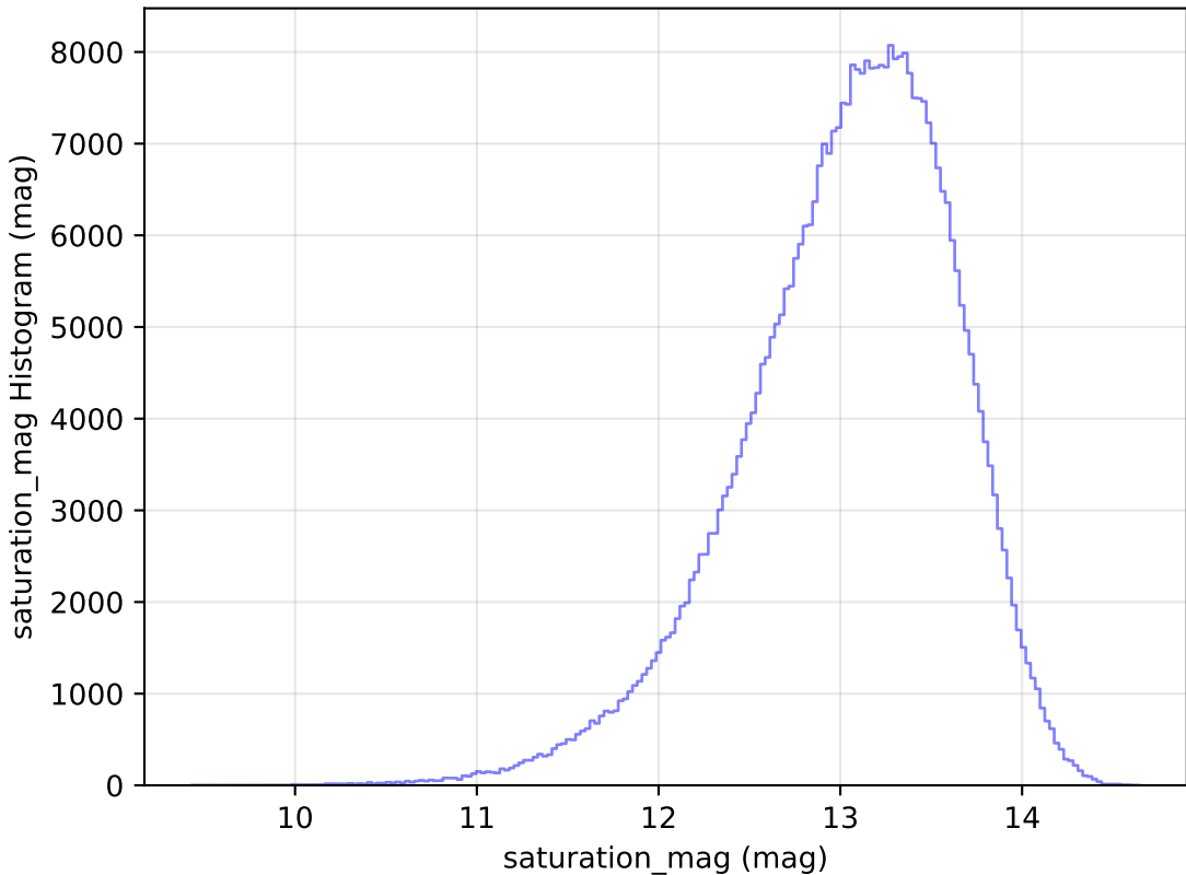
weather_cloudso6v3.4_10yrs WFD y band: saturation_mag Histogram
