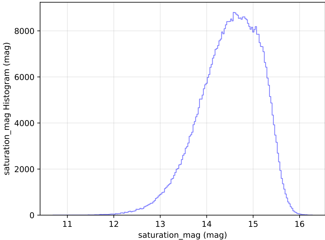
weather_cloudso6v3.4_10yrs WFD r band: saturation_mag Histogram
